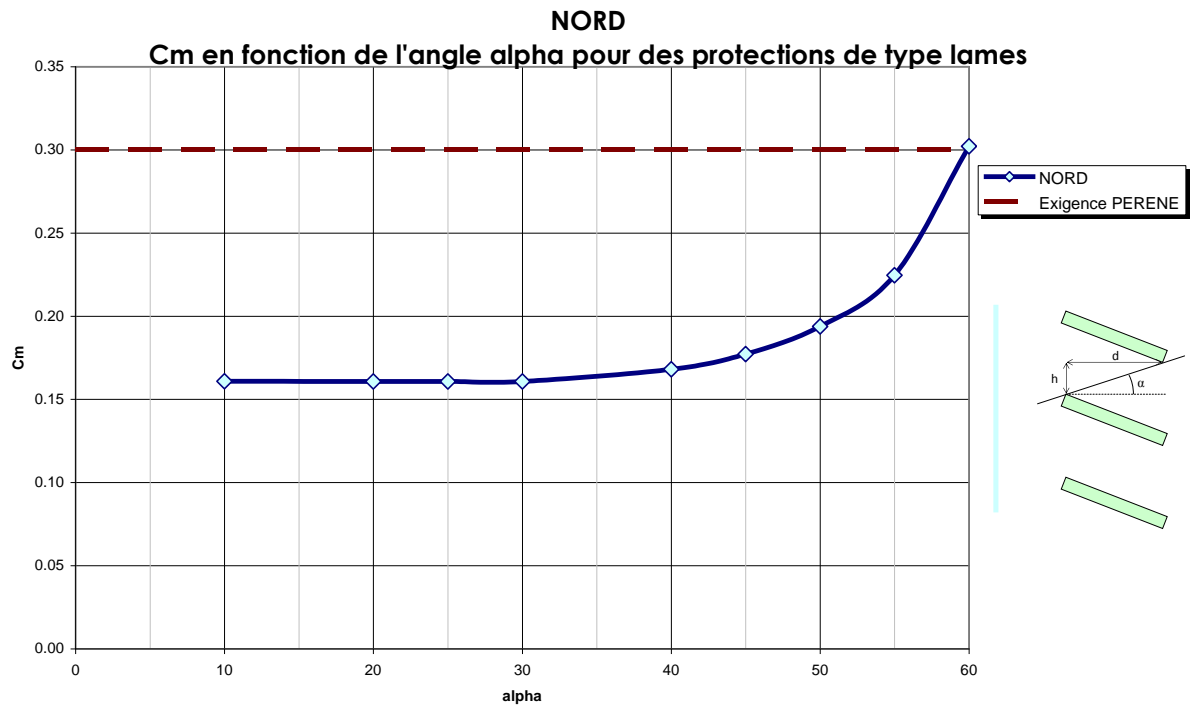
Figure F. 19 : Valeurs de Cm pour des lames pour une orientation NORD
