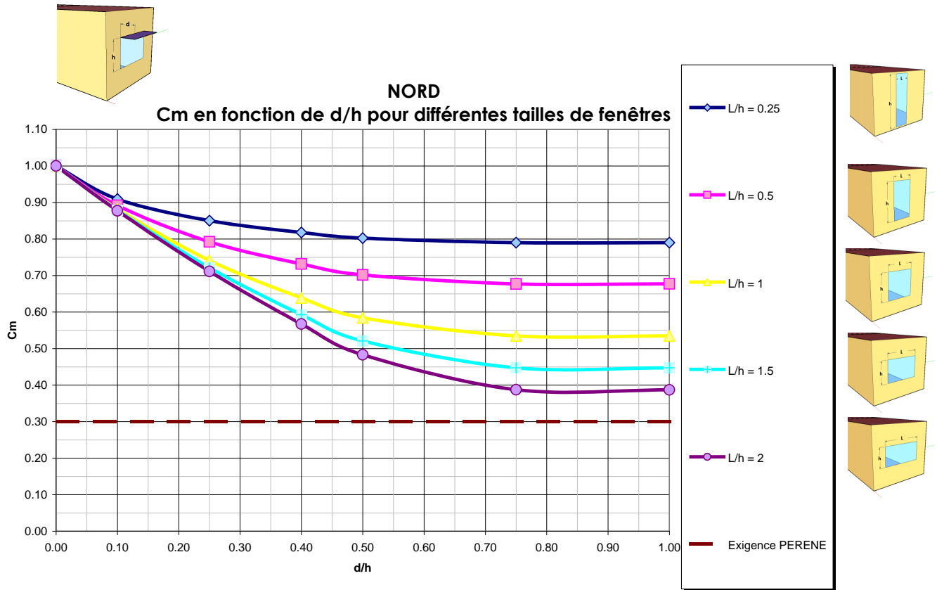
Figure F. 6 : Valeurs de Cm en fonction de d/h quand le rapport L/h varie pour une orientation NORD
