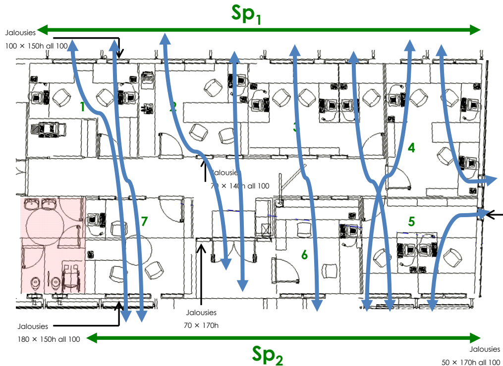
Figure 23 : Calcul de la porosité dans le cas d'un bâtiment de bureaux
