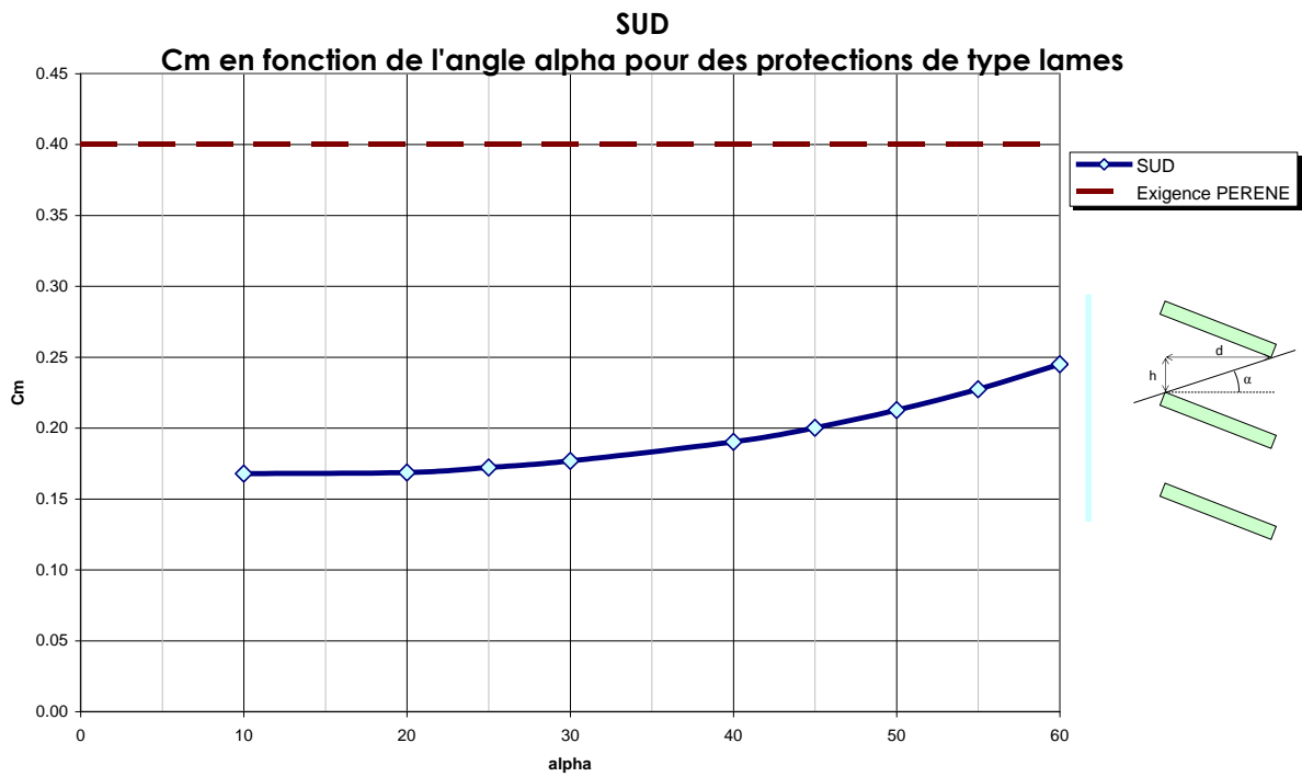
Figure F. 20 : Valeurs de Cm pour des lames pour une orientation SUD
