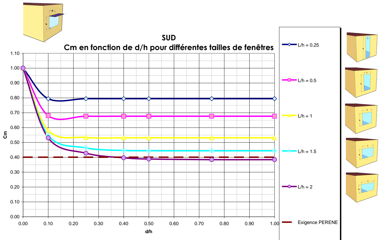
Figure F. 7 : Valeurs de Cm en fonction de d/h quand le rapport L/h varie pour une orientation SUD
