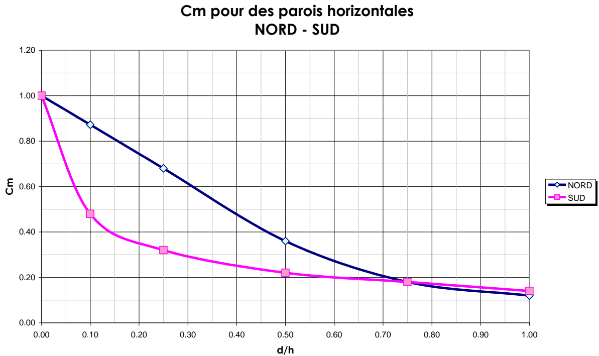
Figure E. 2 : Valeurs de C_m en fonction du rapport d/h pour des parois opaques NORD et SUD
