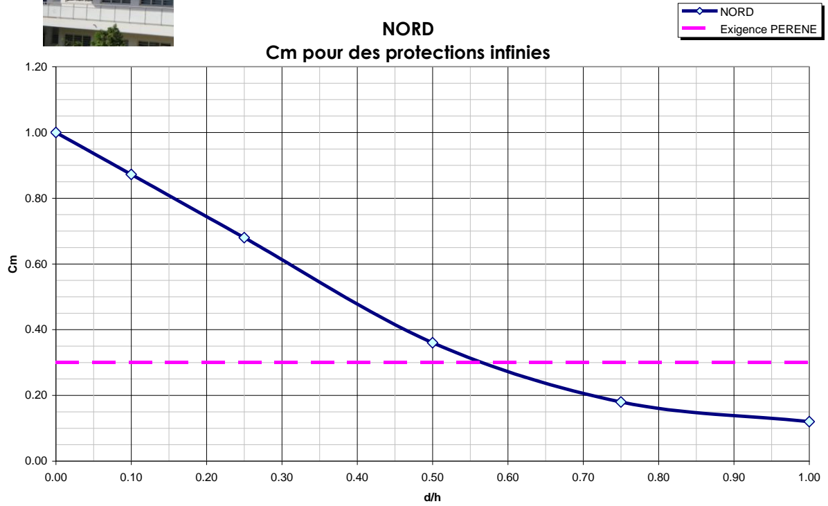
Figure F. 12 : Valeurs de Cm pour un débord infini pour une orientation NORD
