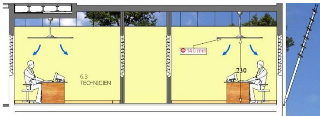
Figure 8 : Implantation des brasseurs d’air dans un bureau
