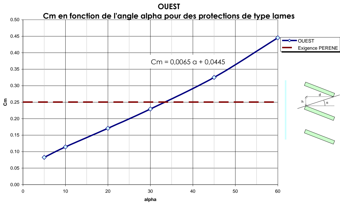
Figure F. 22 : Valeurs de Cm pour des lames pour une orientation OUEST
