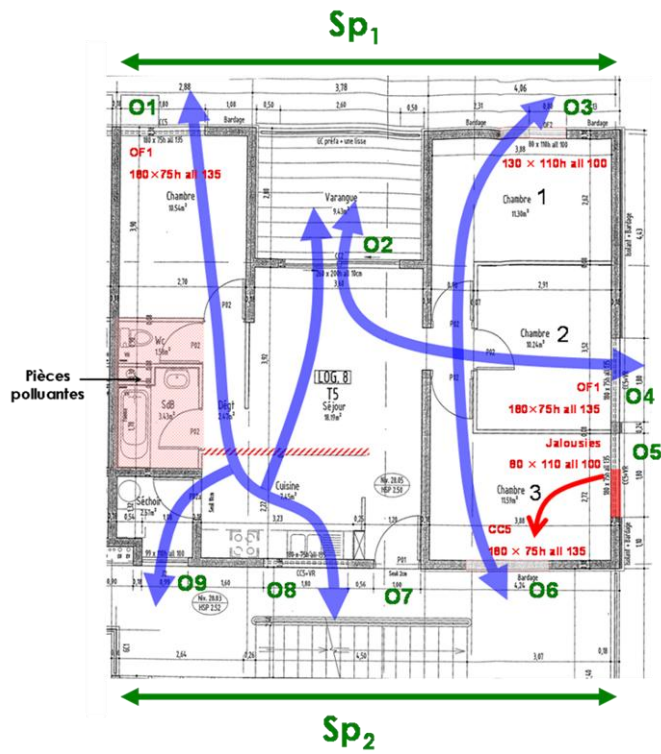
Figure 18 : Modifications apportées pour que les chambres aient une surface d'ouvrant minimale suffisante
