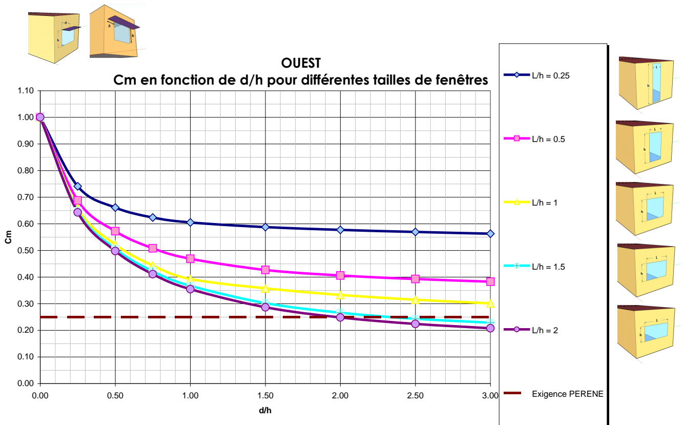
Figure F. 9 : Valeurs de Cm en fonction de d/h quand le rapport L/h varie pour une orientation OUEST
