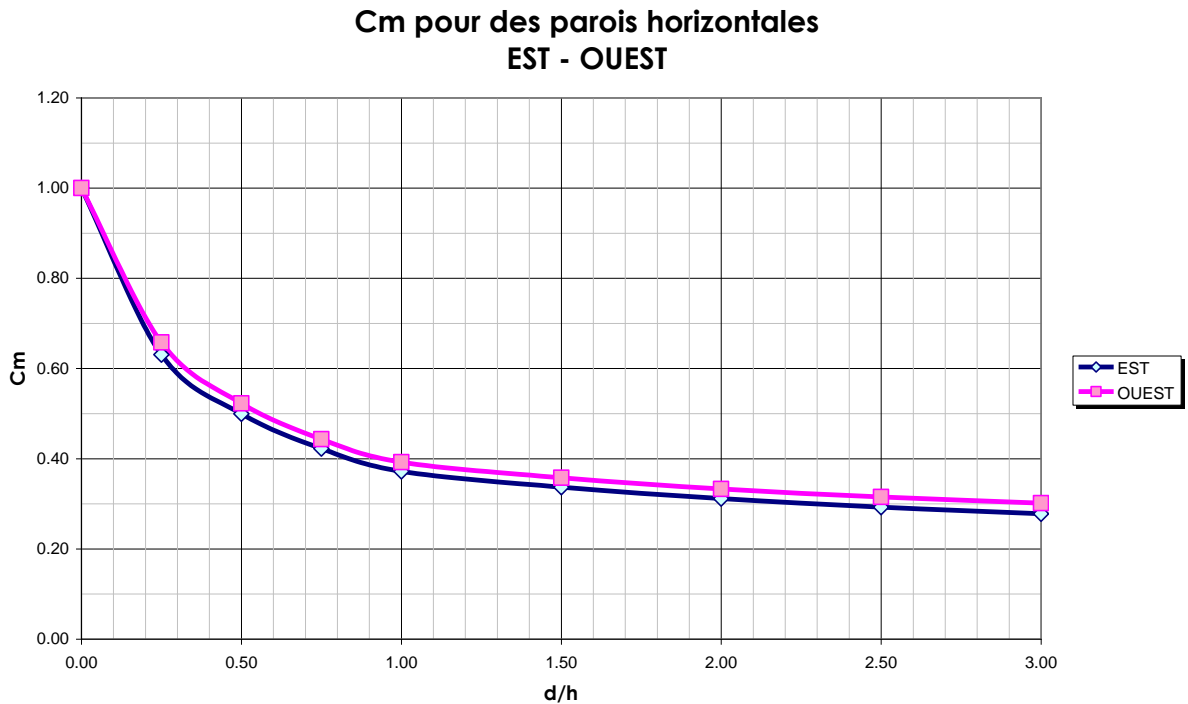
Figure E. 3 : Valeurs de C_m en fonction du rapport d/h pour des parois opaques EST et OUEST
