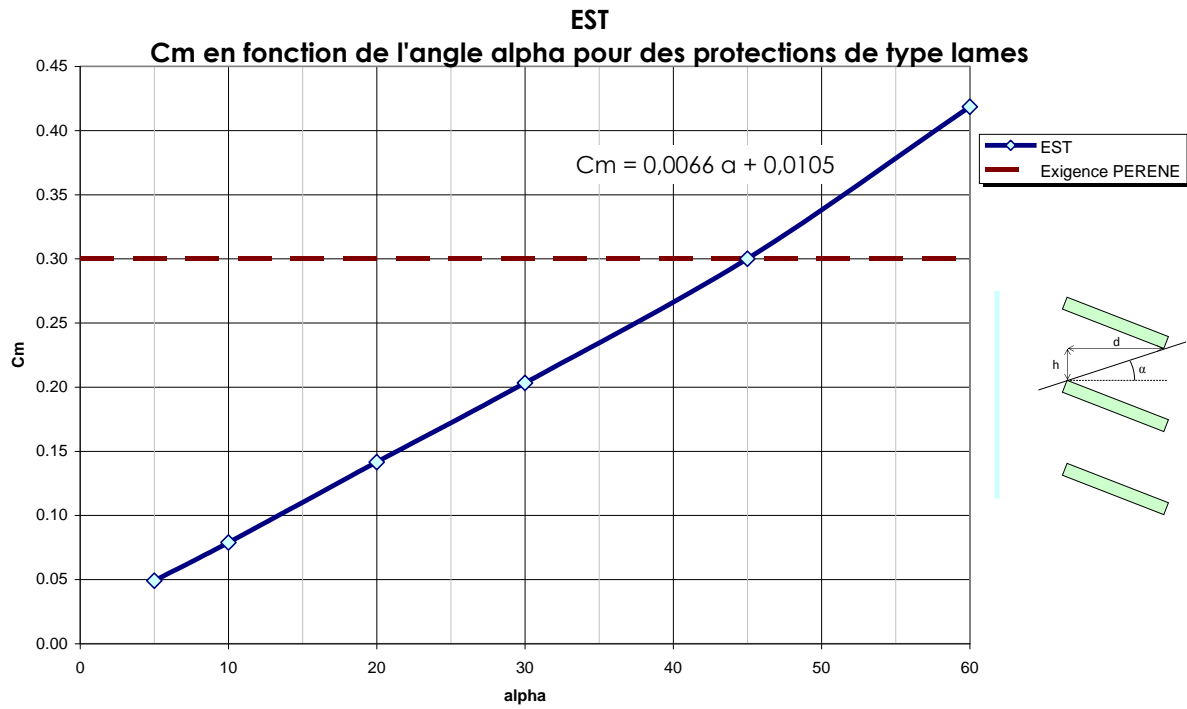
Figure F. 21 : Valeurs de Cm pour des lames pour une orientation EST
