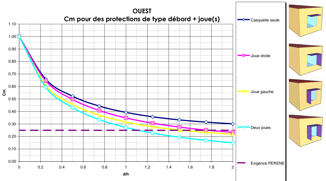
Figure F. 17 : Valeurs de Cm pour des solutions de type débord + joue(s) pour une orientation OUEST
