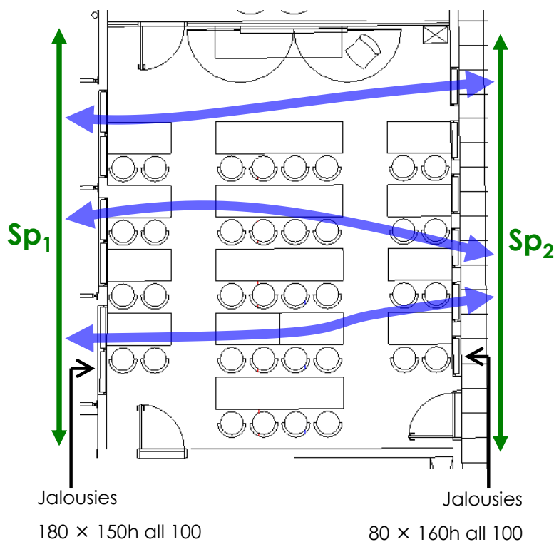
Figure 22 : Calcul de la porosité dans le cas d'une salle de classe
