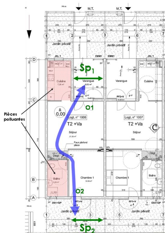
Figure 14 : exemple de logement T2 est bien traversant.
