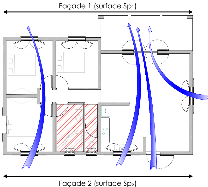
Figure 5 : Ventilation traversante via 2 façades opposées
