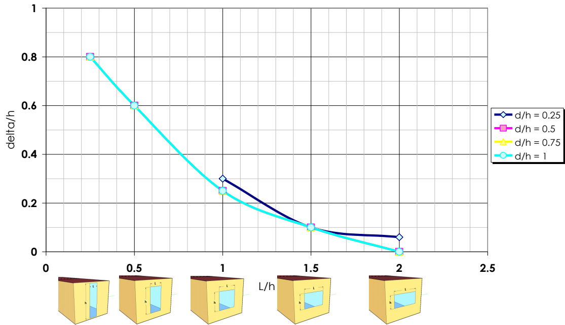
Figure F. 11 : Valeurs du rapport \delta/h en fonction de L/h pour avoir C_m = 0,40 pour une orientation SUD
