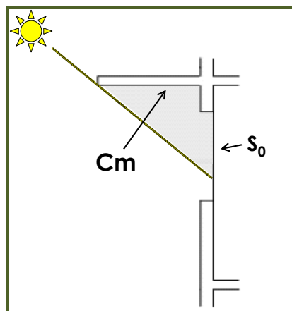
Figure 6 : Coefficient d'ensoleillement
