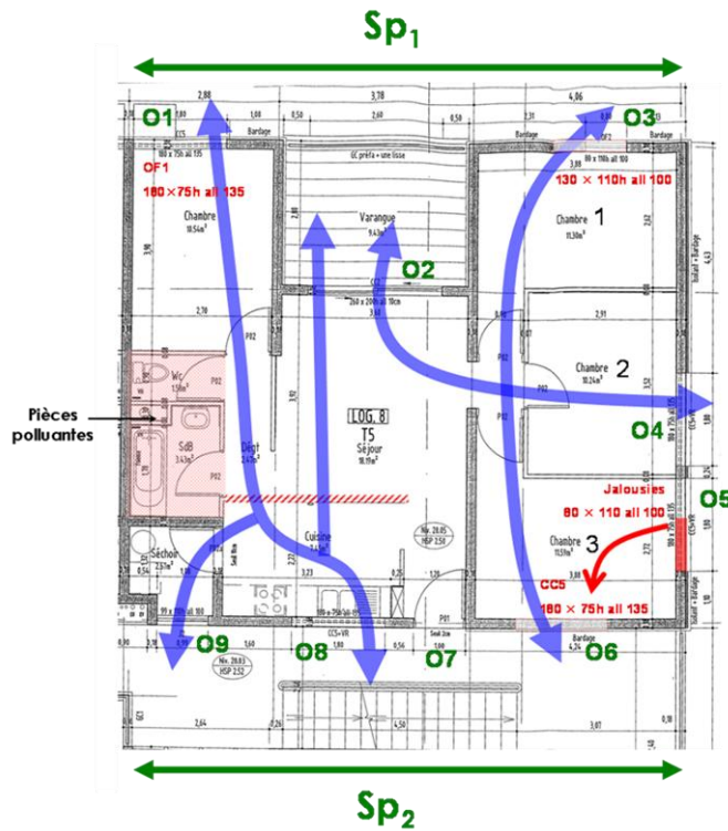
Figure 17 Modifications apportées pour obtenir la porosité demandée du T5 en Z1
