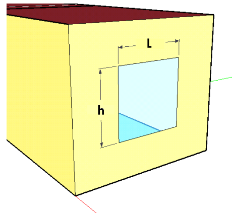
Figure F. 2 : Définition du rapport L/h d'une baie
