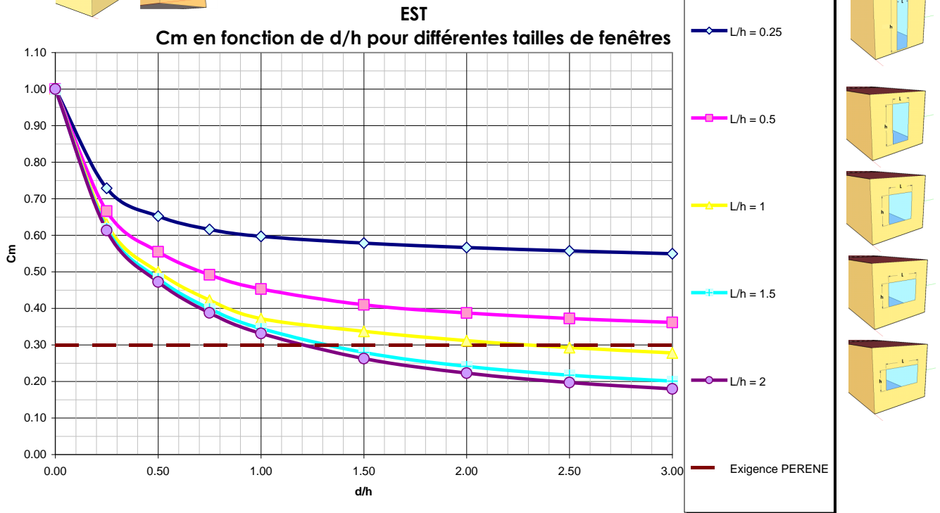
Figure F. 8 : Valeurs de Cm en fonction de d/h quand le rapport L/h varie pour une orientation EST
