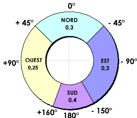
Figure 7 : Définition des orientations pour les zones 1-2-3 7
