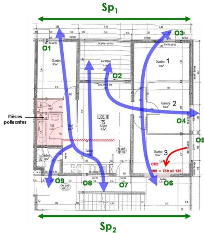
Figure 16 : Modifications apportées pour obtenir le côté traversant d'un T5 en Z1
