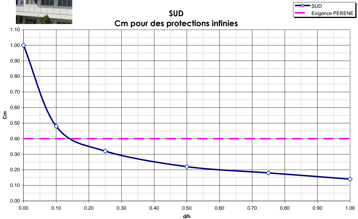
Figure F. 13 : Valeurs de Cm pour un débord infini pour une orientation SUD
