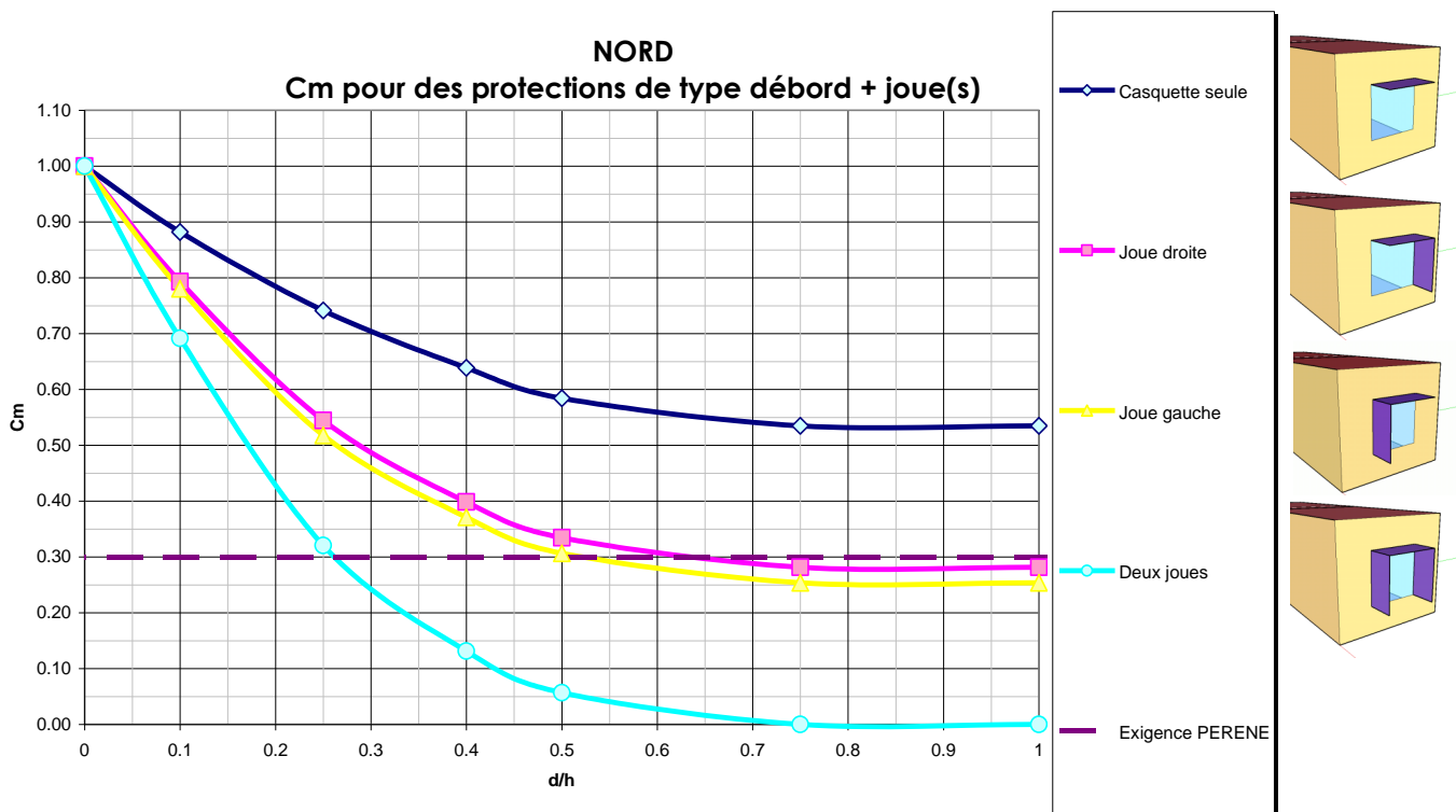
Figure F. 14 : Valeurs de Cm pour des solutions de type débord + joue(s) pour une orientation NORD
