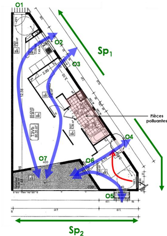
Figure 21 : Modification apportée pour avoir un logement traversant
