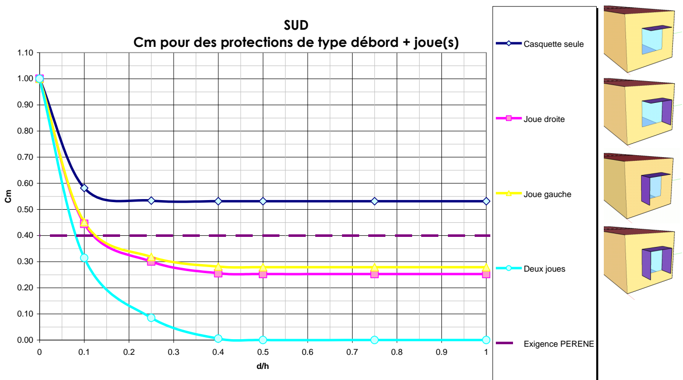
Figure F. 15 : Valeurs de Cm pour des solutions de type débord + joue(s) pour une orientation SUD
