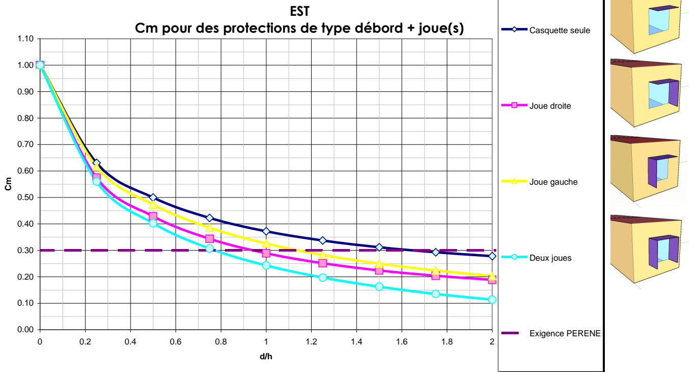
Figure F. 16 : Valeurs de Cm pour des solutions de type débord + joue(s) pour une orientation EST
