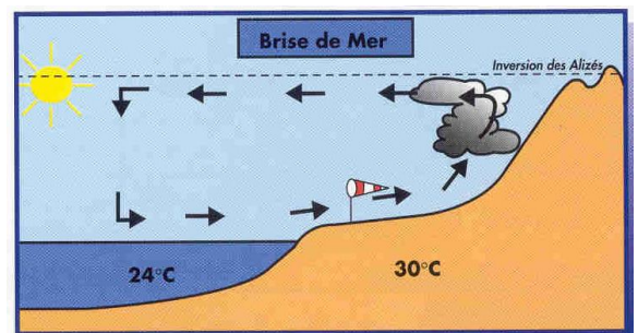
Figure 12 : Brise de mer Source atlas météo France
