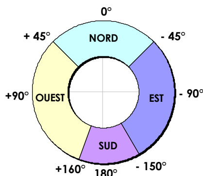
Figure : Définition des orientations des baies et parois opaques en fonction de l'azimut
