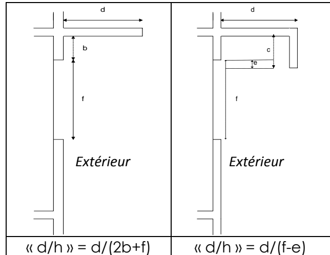
Figure F. 1 : Définition du « d/h » équivalent
