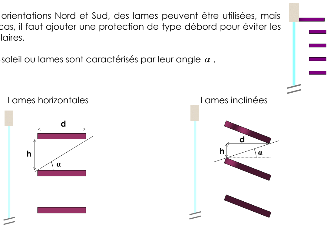
Figure F. 18 : Définition de \alpha pour des lames horizontales et inclinées
