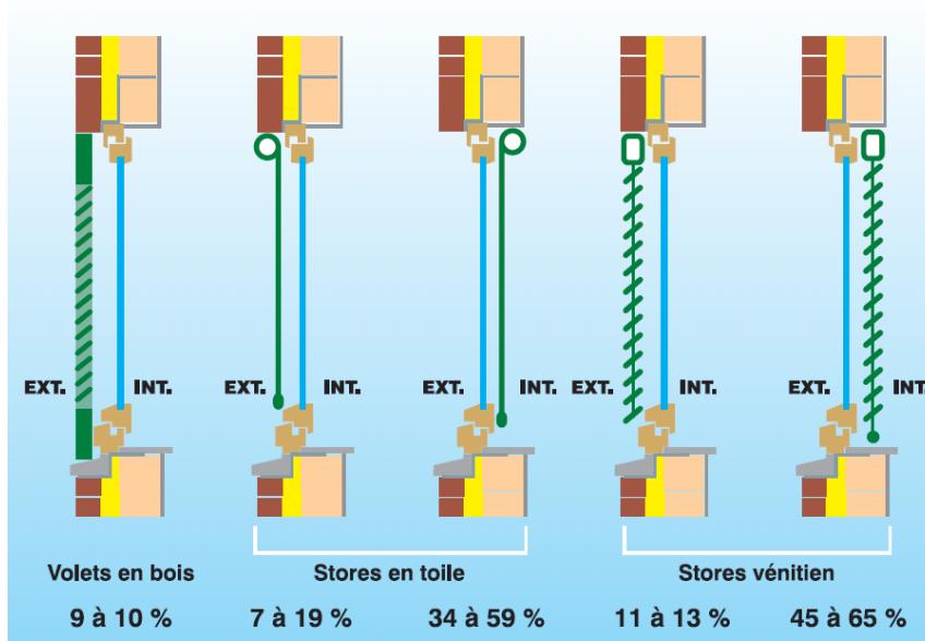
Figure F. 23 : Facteurs solaires de différentes protections solaires pour un vitrage simple [Liébard 2005]
