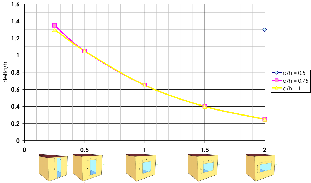
Figure F. 10 : Valeurs du rapport \delta/h en fonction de L/h pour avoir C_m = 0,30 pour une orientation NORD
