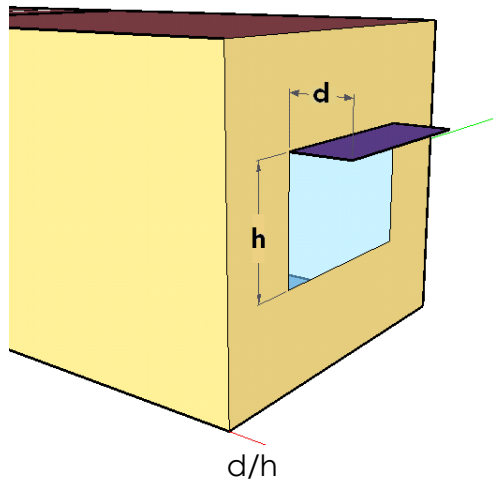
Figure F. 1 : Définition du « d/h » équivalent
