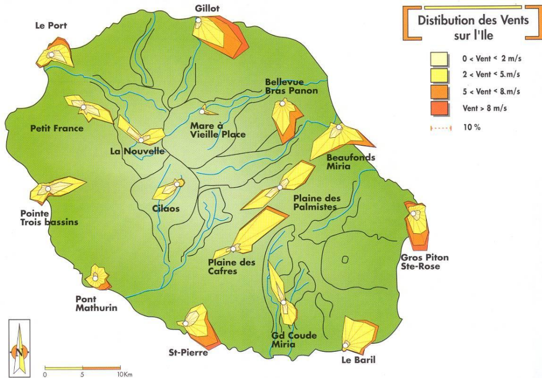
Figure 9 : Cartographie Réunion Rose des vents – Source Météo France
