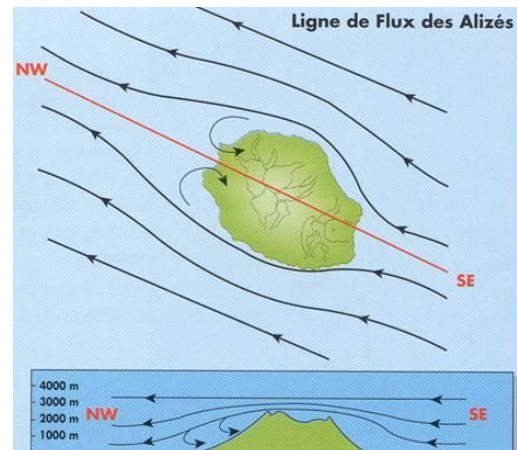
Figure 11 : direction des alizés Source atlas météo France
