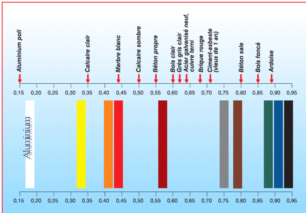
Figure 24 : Coefficients d'absorption a pour différents matériaux et différentes couleurs. Source : (Liébard 2005)
